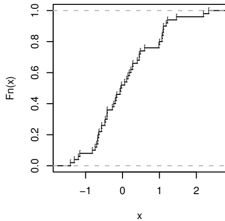
ecdf(norm50)
