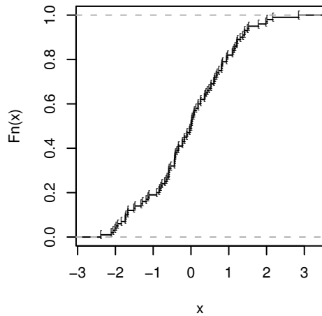
ecdf(norm100)
