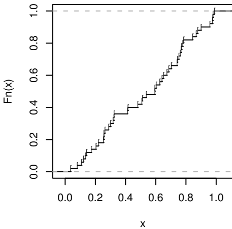
ecdf(unif50)
