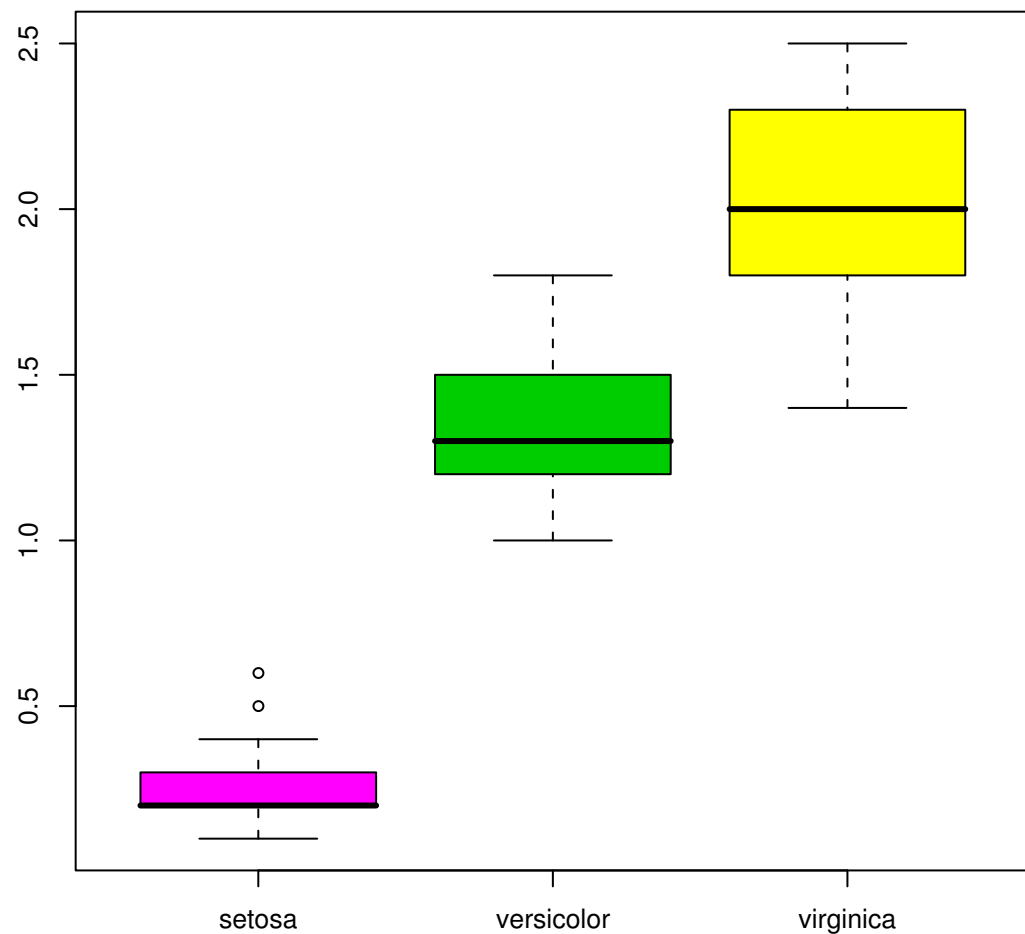
Petal Width
