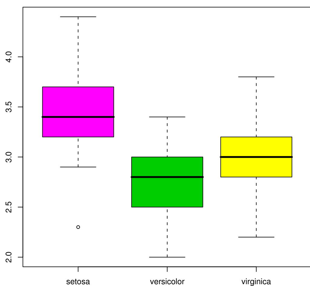
Sepal Width
