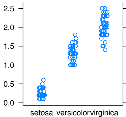
Petal Width
