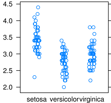
Sepal Width
